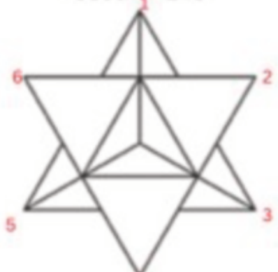
Merkaba
